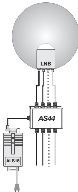
Percorso alimentazione LNB
