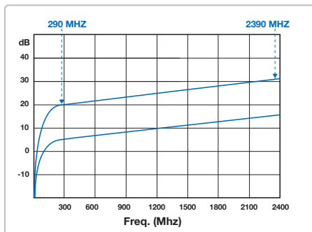
Pegeldämpfungssteller
